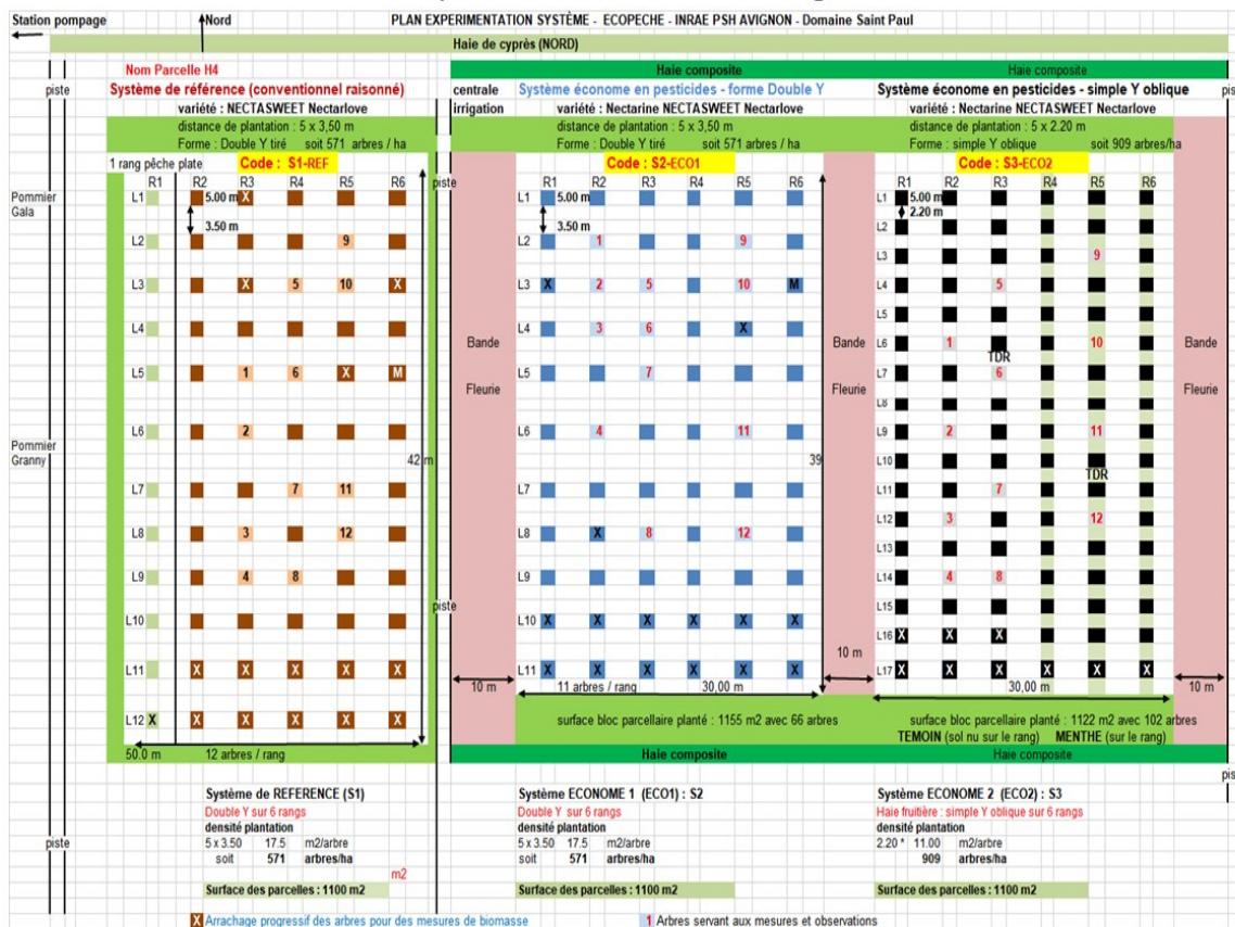
Plan du dispositif EcoPêche2 INRAE site Avignon
